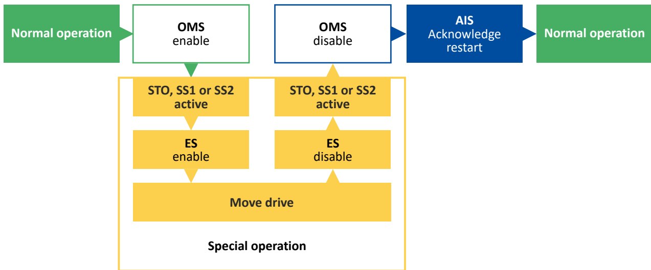
Fig. 19: OMS function
