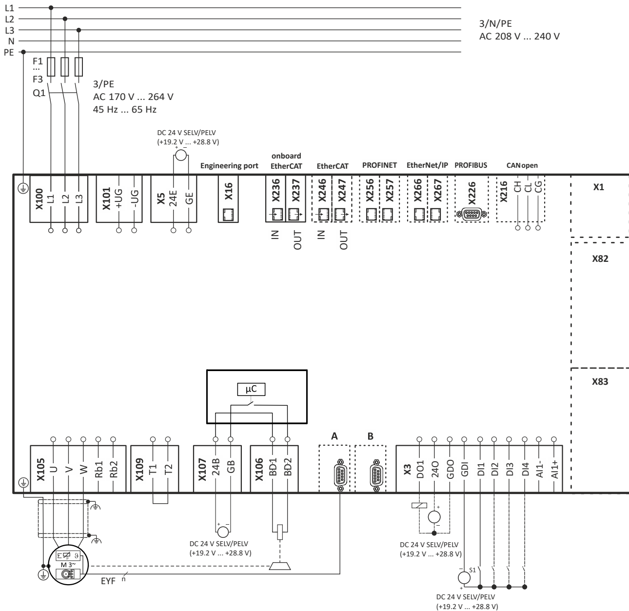
Fig. 3: Wiring example
