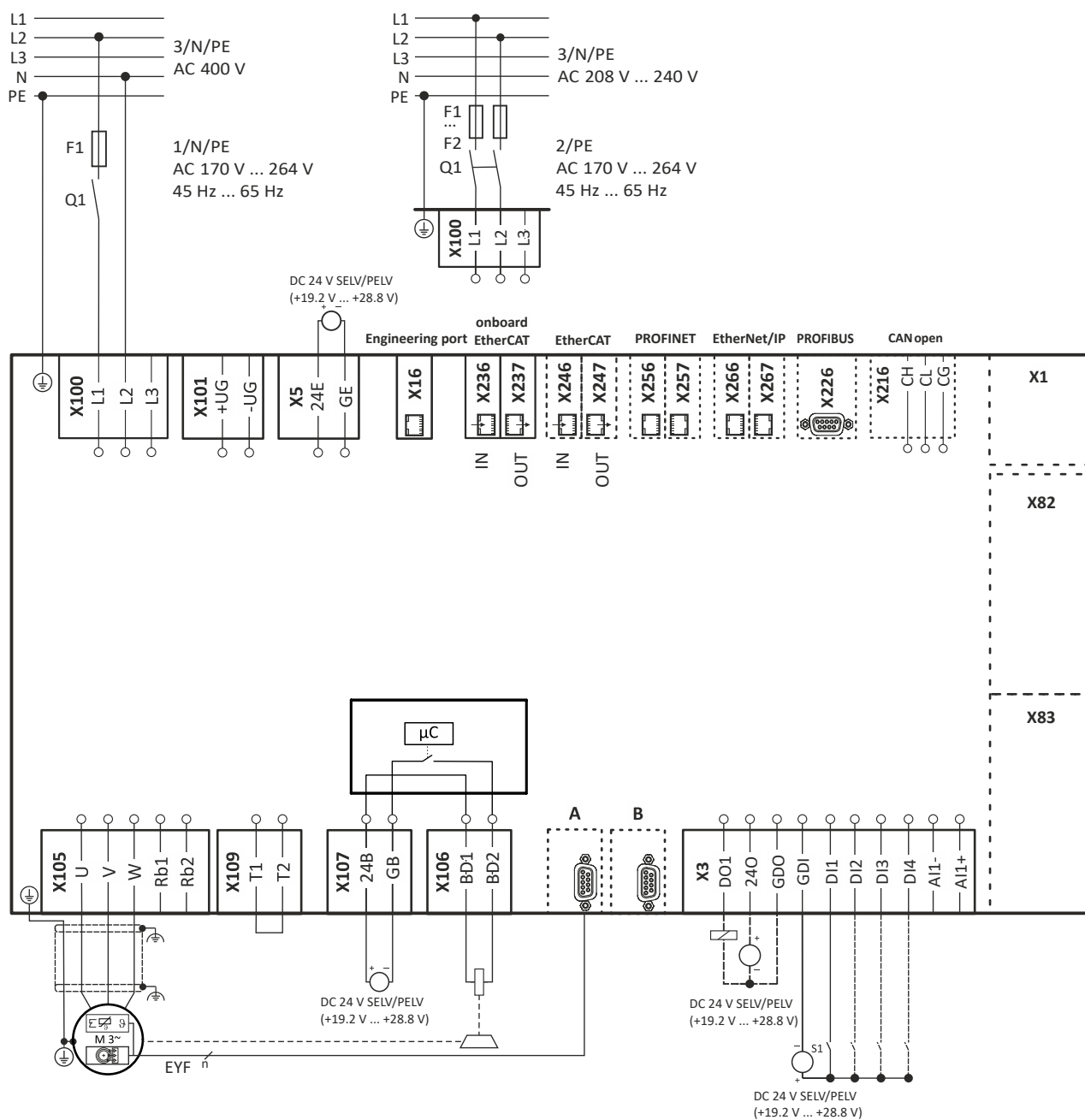
Fig. 2: Wiring example
