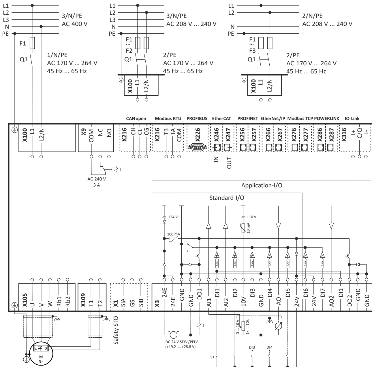
Fig. 3: Wiring example
