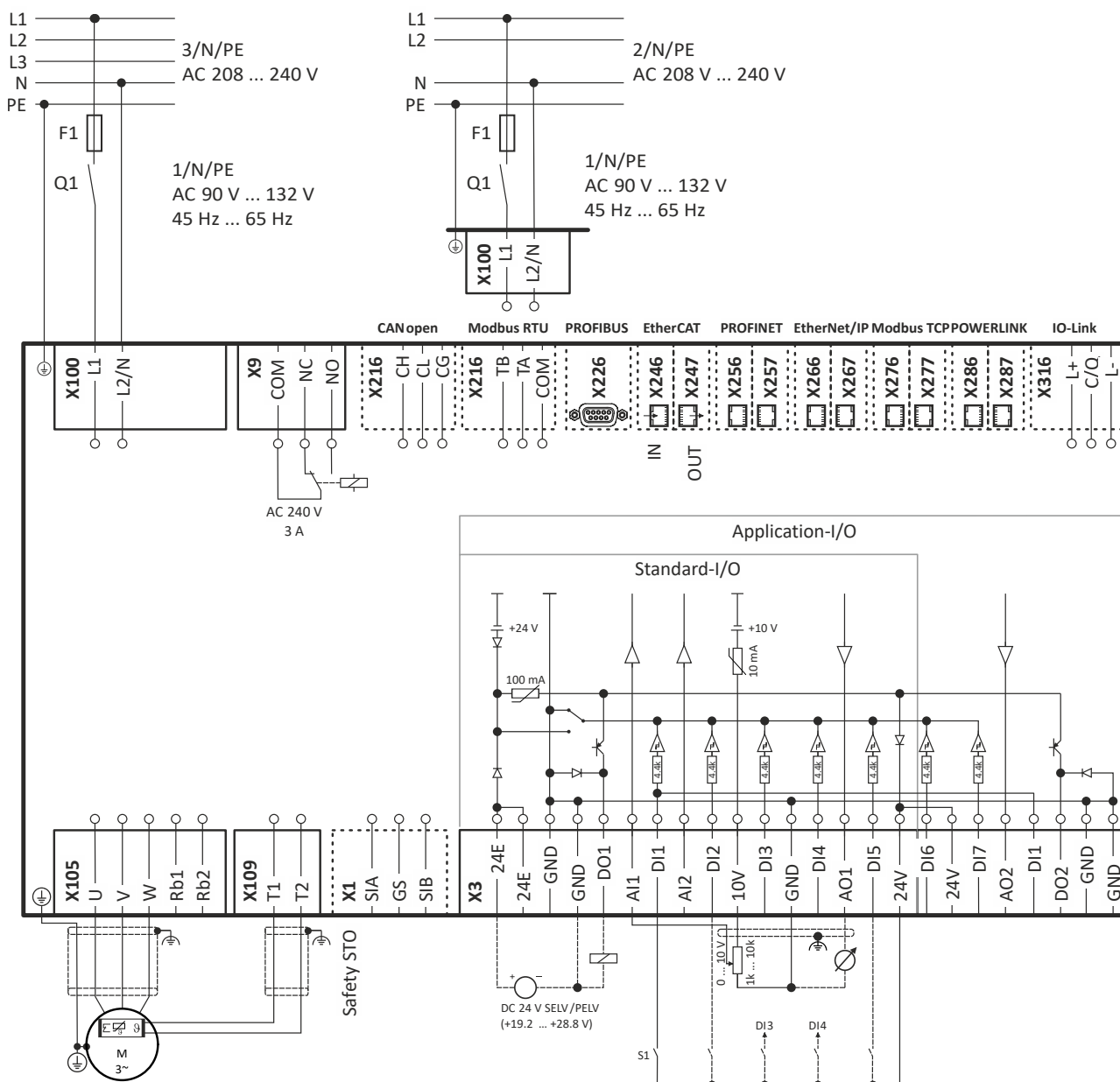
Fig. 2: Wiring example
