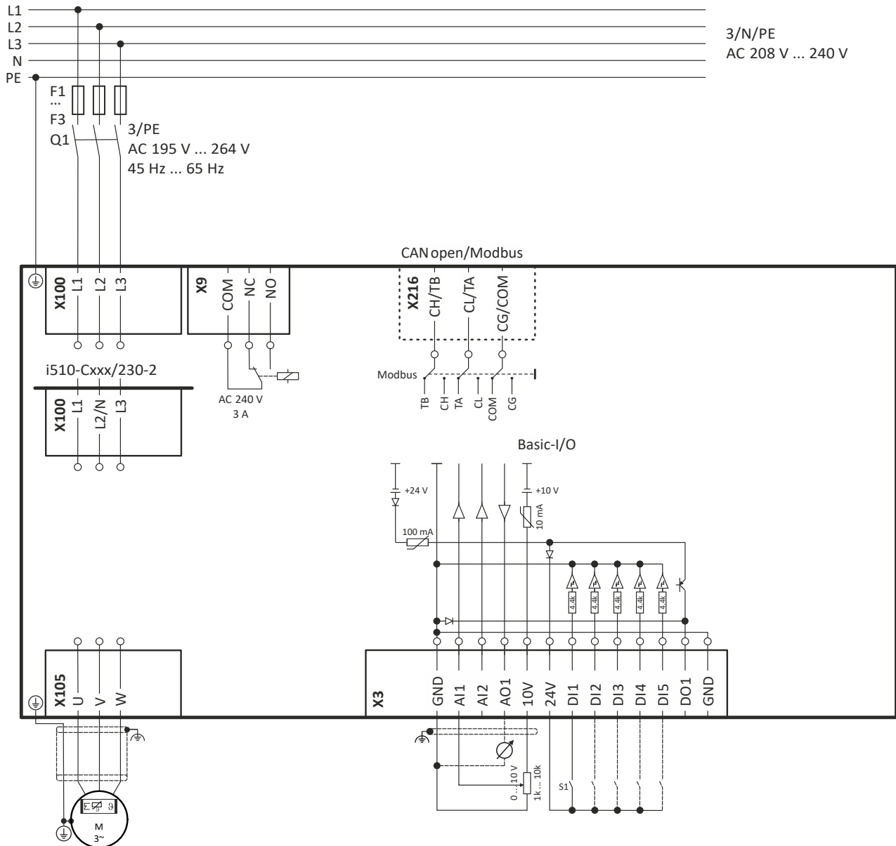
Fig. 4: Wiring example
